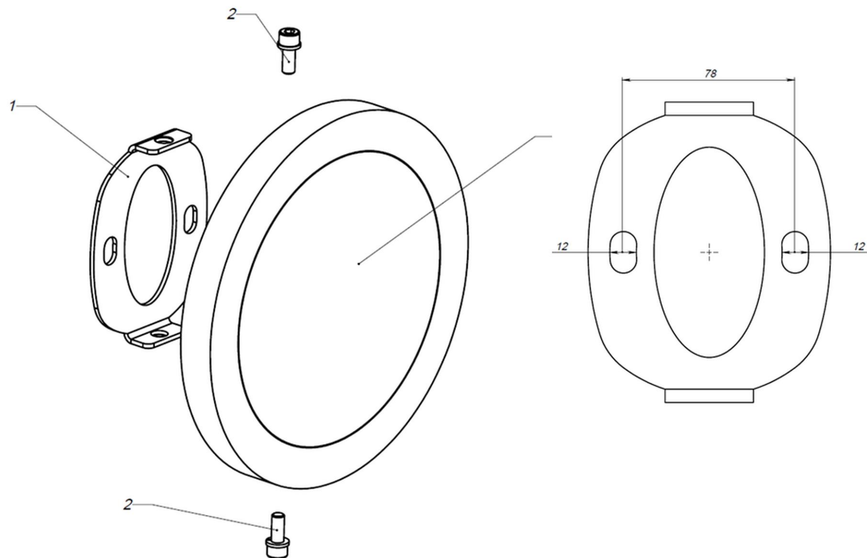
Рисунок 3. Монтажная инструкция
